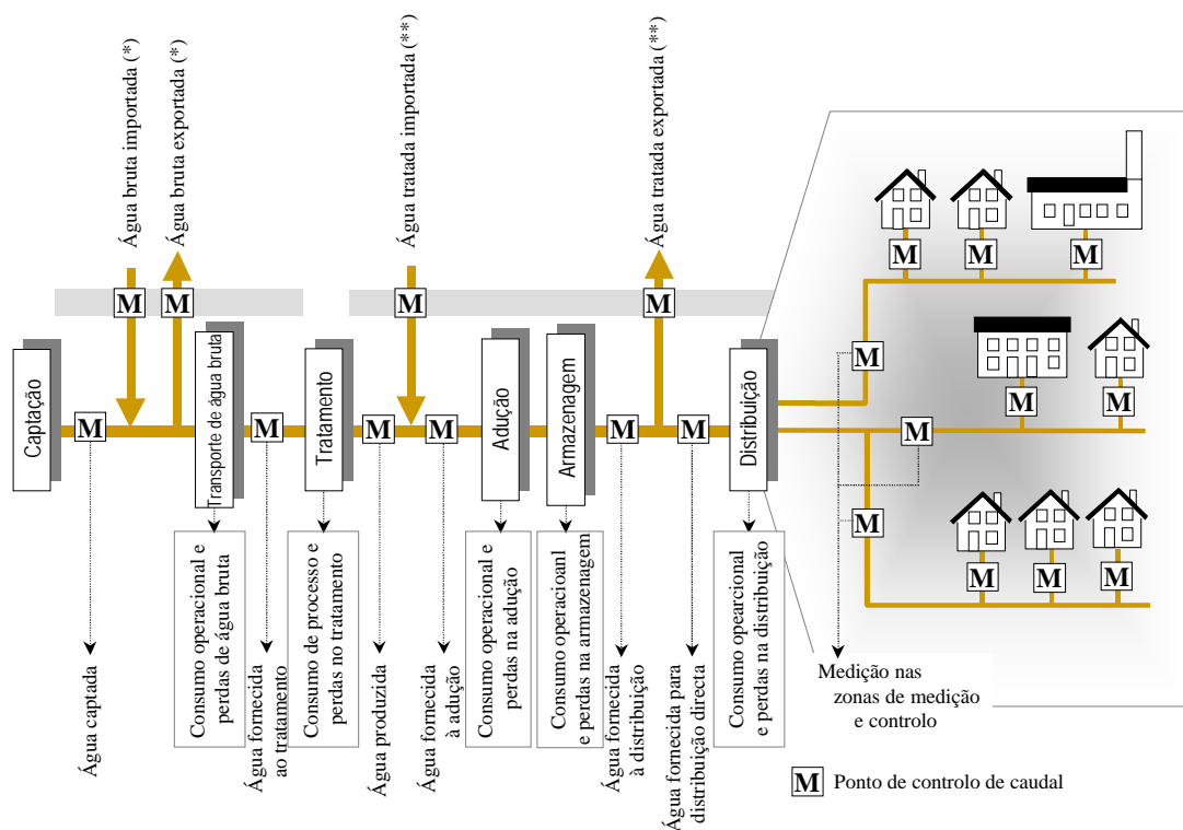
Figura 1 – Principais elementos dos sistemas de abastecimento de água, com identificação dos componentes do balanço hídrico e localização dos pontos de controlo de caudal
