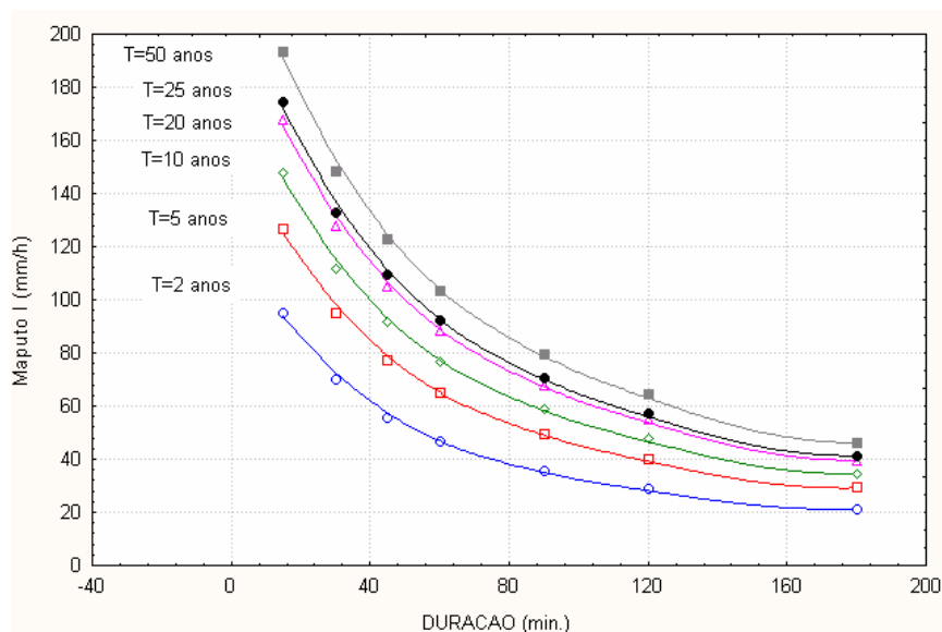
Expressão gráfica das curvas I-D-F para Maputo
